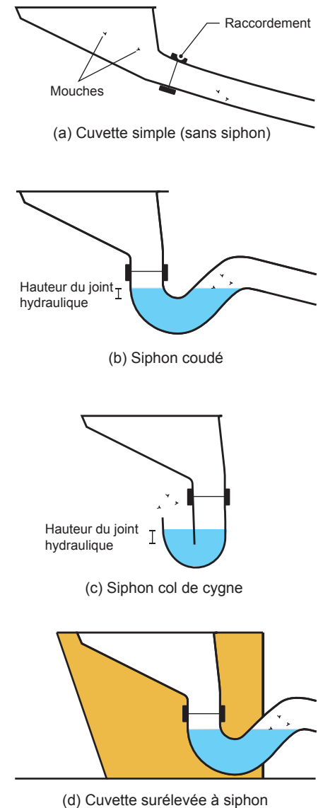
Figure 2. Modèles de cuvette
