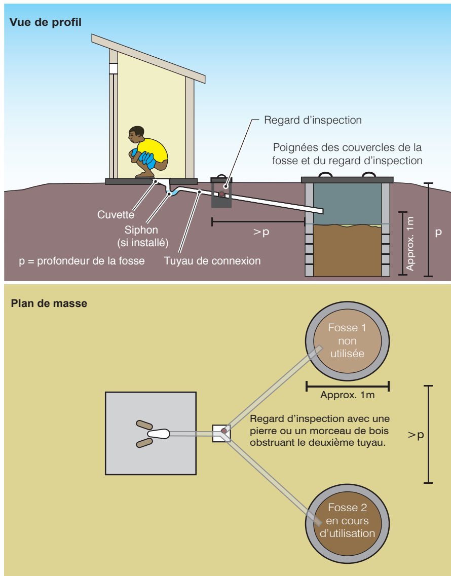
Figure 4. Une latrine à eau avec fosse sous la superstructure
