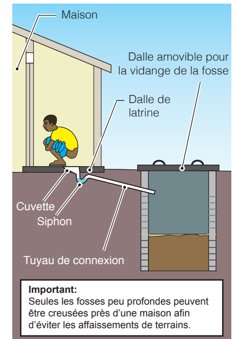
Figure 1. Une latrine à eau avec fosse déportée
