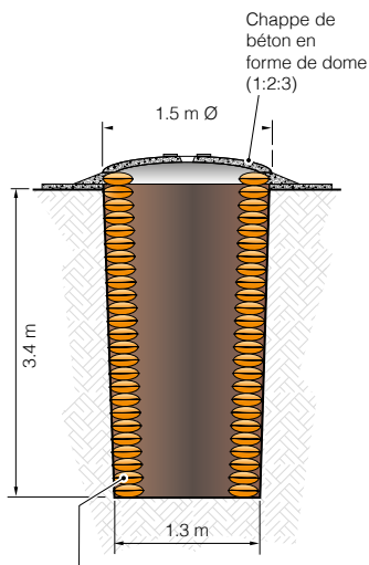
Revêtement avec des sacs de sable 142 mm d'épaisseur
