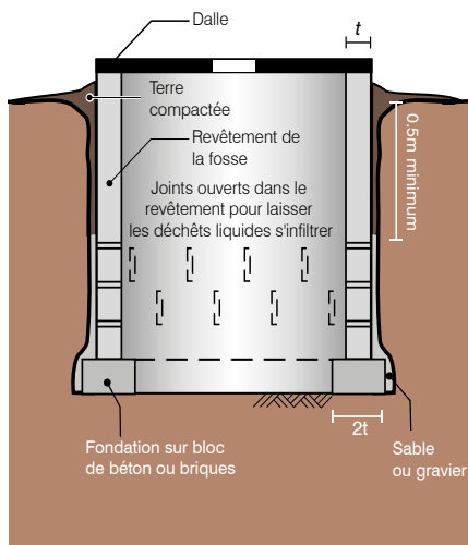
Figure 2. Détails de la construction d'une fosse peu profonde avec revêtement
